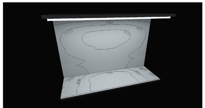
OPSLM-A860・D 棚W900mm×H600mm×D300mmに860mmのモジュール取付時
