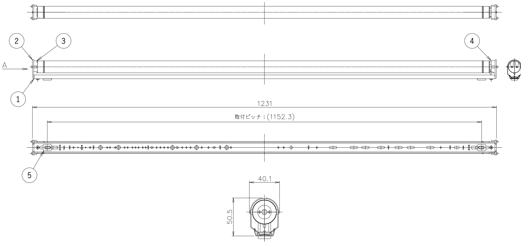
A矢視図
