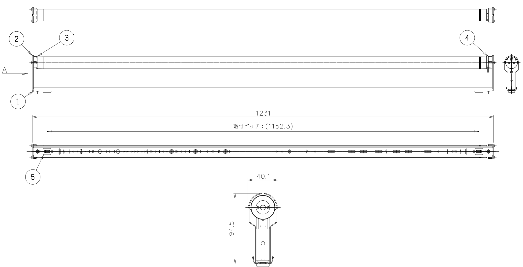
A矢視図
